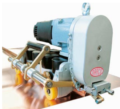
Der Dachfalzschließer K9-1 mit Duo-Funktionsschalter K9-1-DF.
