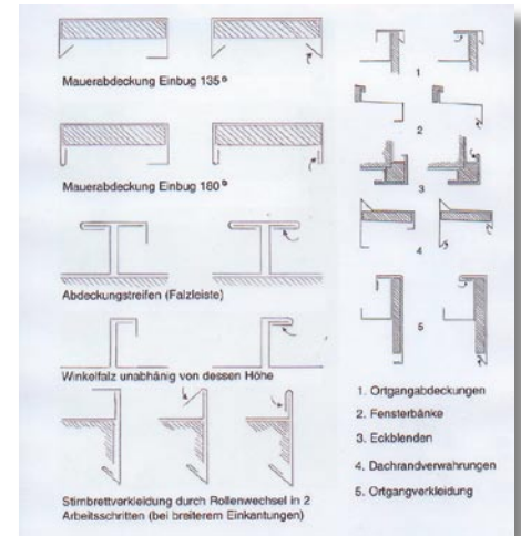
Beispiele für den Einsatz des Rollformers.
